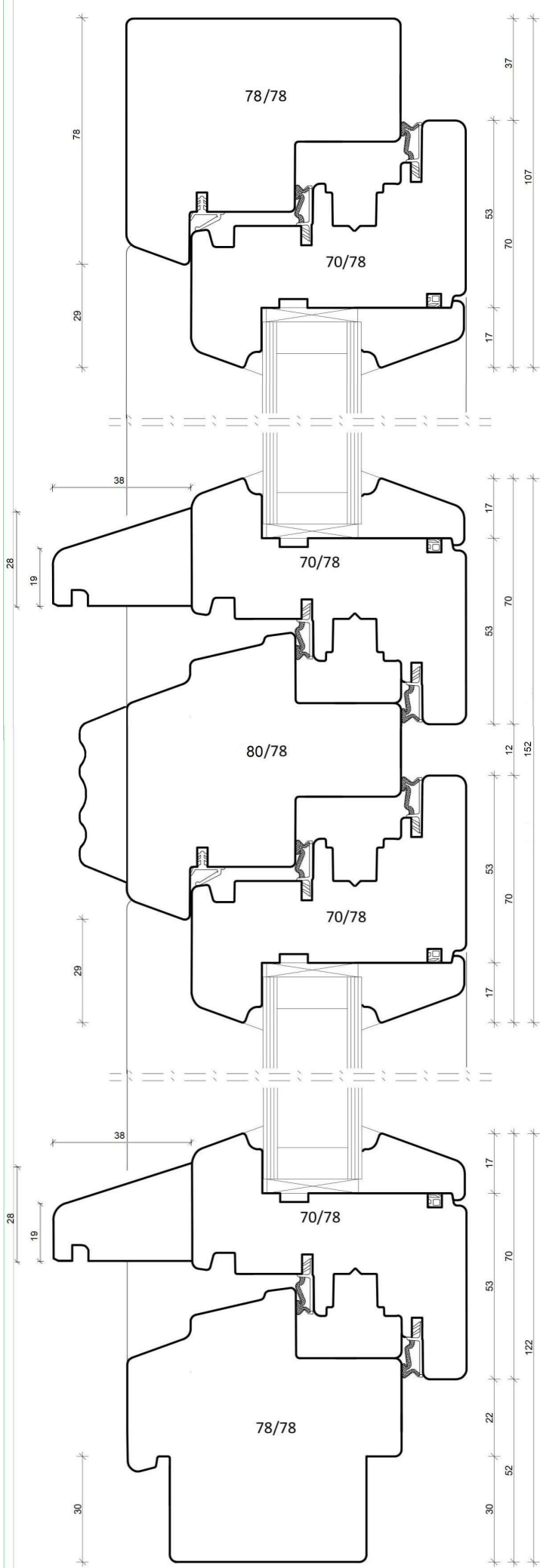
VERTIKALSCHNITT DENKMAL IV 78 - 17
